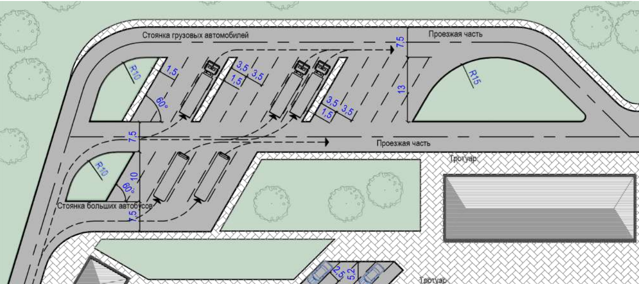
ПАРКОВКИ И СТОЯНКИ ПОД УГЛОМ 45 ГРАДУСОВ
