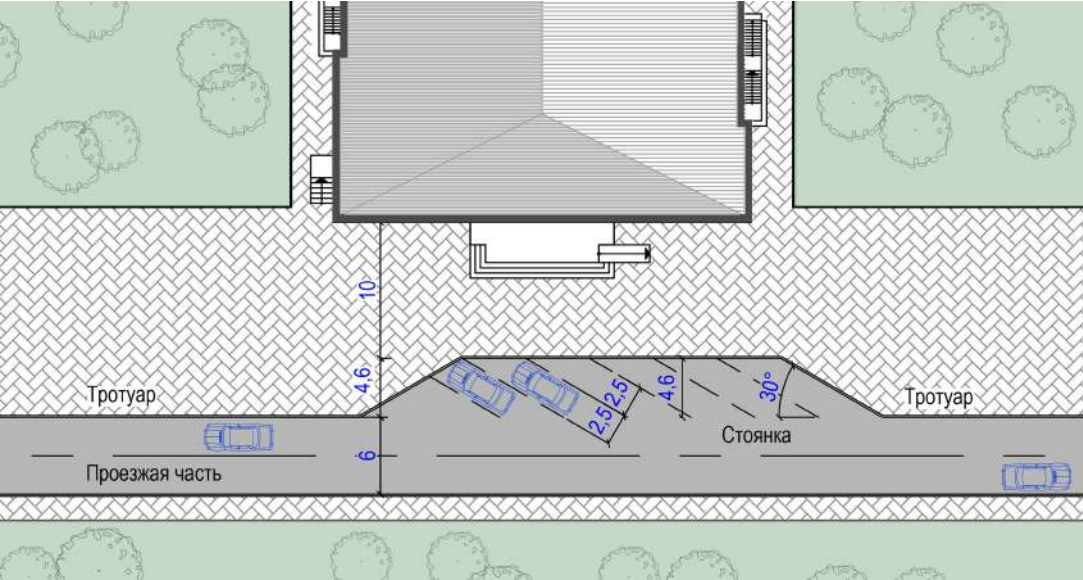
ПАРКОВКИ И СТОЯНКИ ПОД УГЛОМ 30 ГРАДУСОВ
