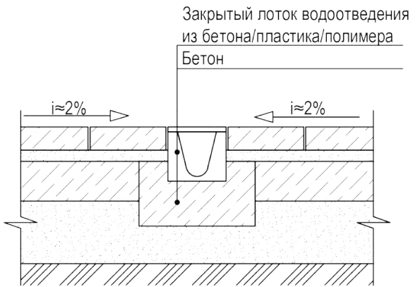
3.20 Схема устройства закрытого лотка водоотведения
