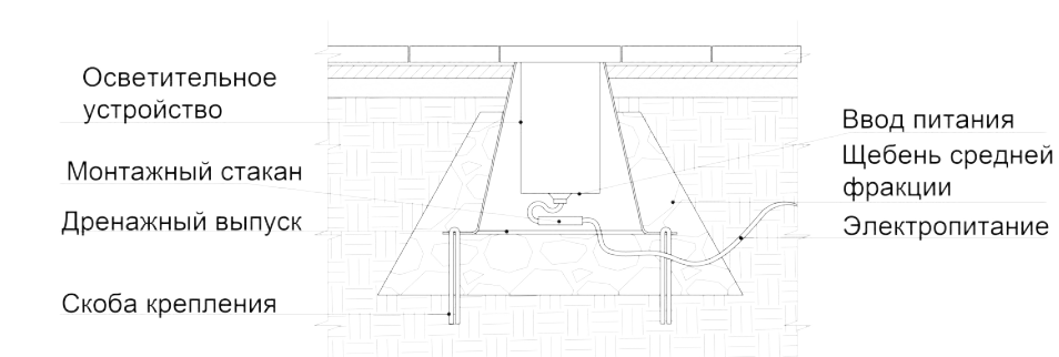
3.18 Схема установки светильника в покрытие
