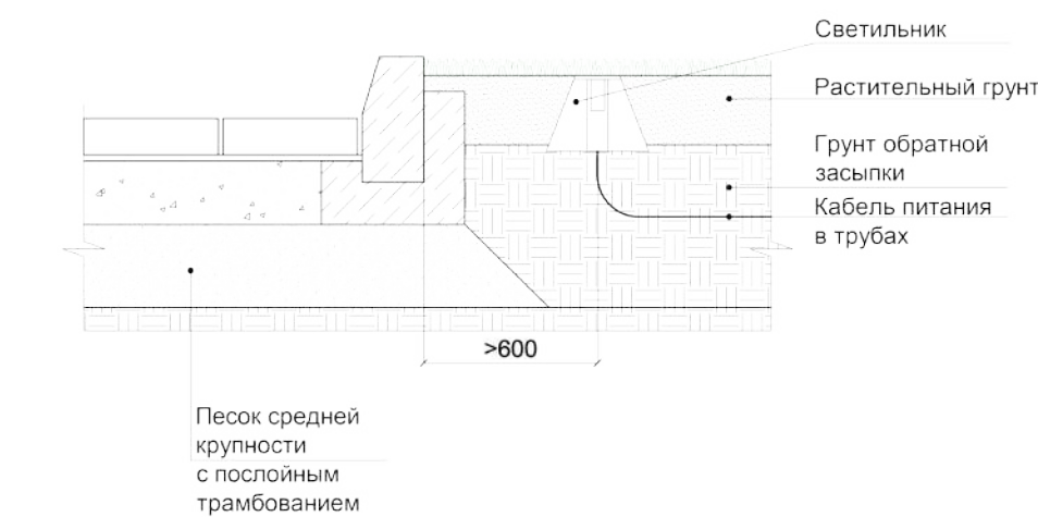
3.19 установка светильника в грунт
