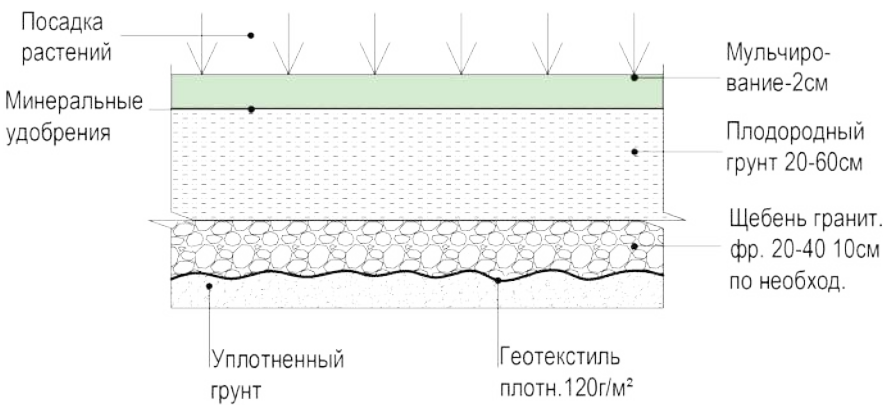
3.10 Схема устройства газона
