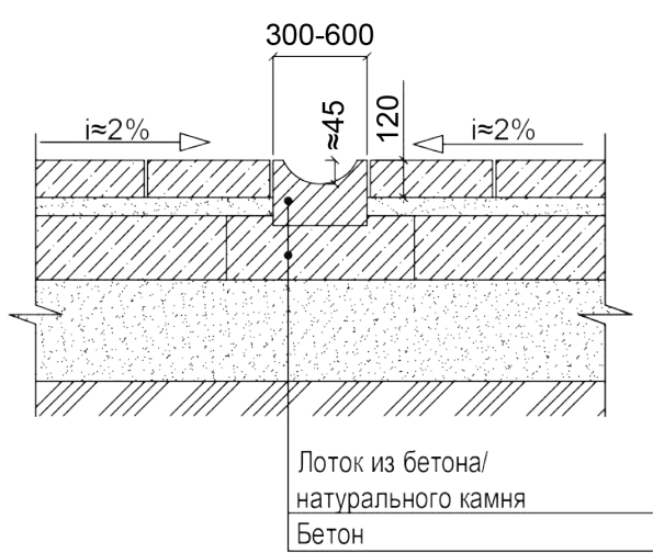
3.21 Схема устройства открытого лотка водоотведения
