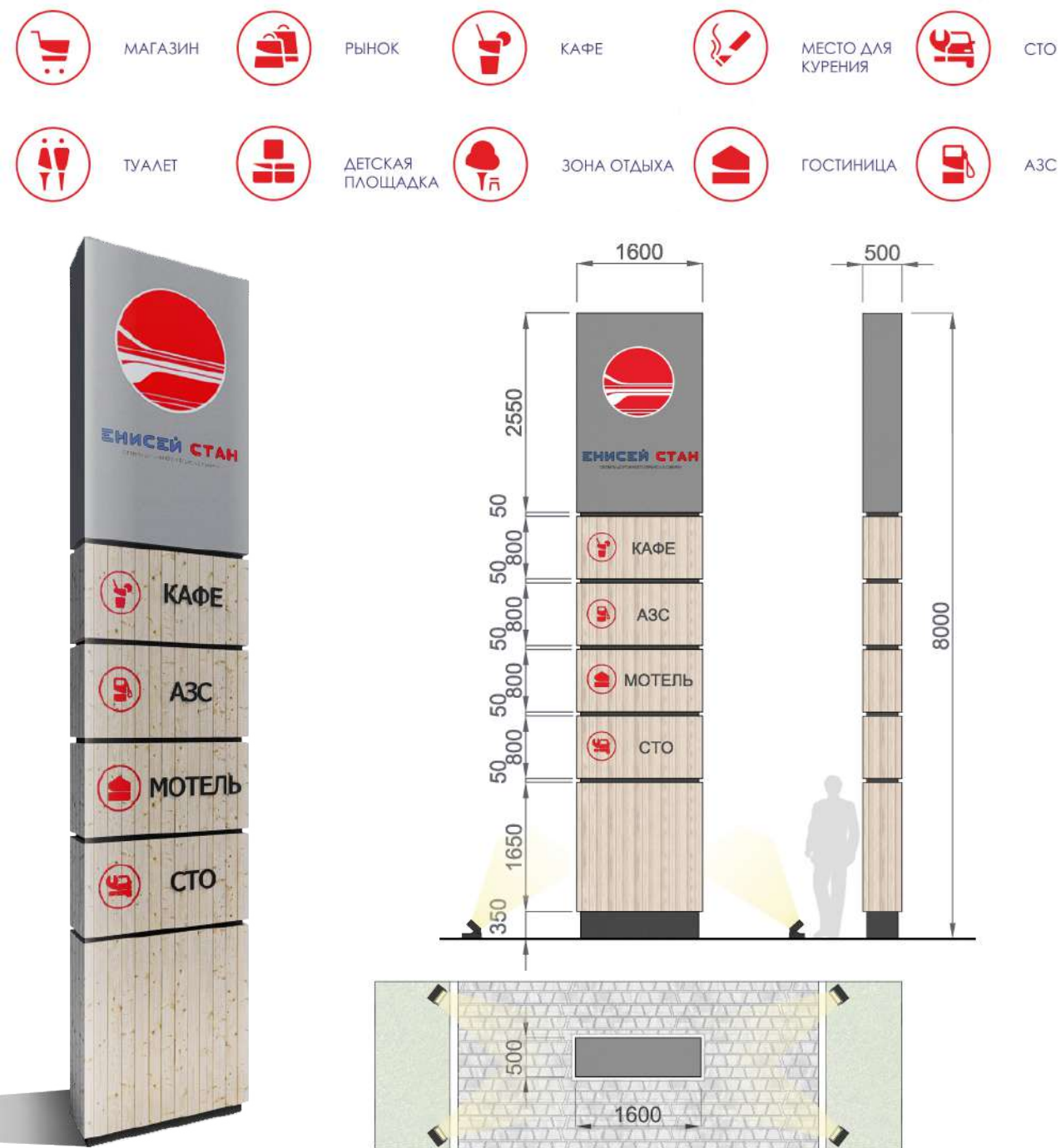
Пример стелы (конструктивное решение, вариативность заполнения модулей стелы, пиктограммы для типов ОДС)
