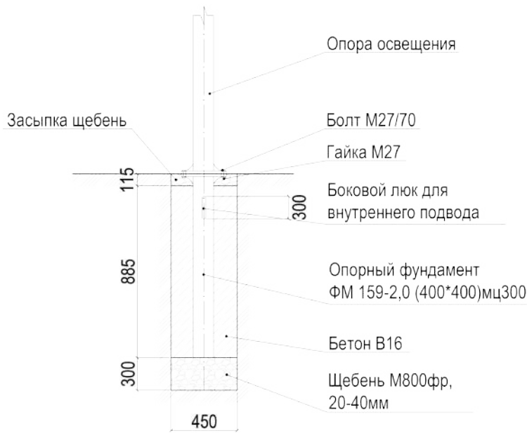
3.16 Схема монтажа опоры освещения
