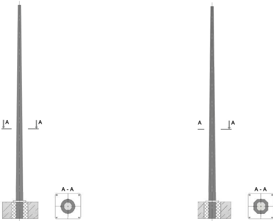
Металлическая круглоконическая опора
